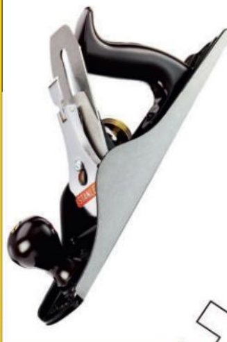
ΡΟΚΑΝΙ BAILEY JACK N° 5 Επαγγελματικό πλήρως ρυθμιζόμενο ροκάνι. Ροδέλα ρύθμισης βάθους κοπής, μοχλός στρέψης, κοχλίας κίνησης βάσης που επιτρέπει την αύξηση ή τη μείωση του αυλακιού. Επιχρωμιωμένο στοπ. Φινίρισμα από μαύρη λάκα. Χυτοπρεσσαριστή βάση, ρεκτιφιαρισμένη στις 3 πλευρές. Λαβή από συνθετικό υλικό. Δέχεται λάμες 0-12-313, 1-12-313.
